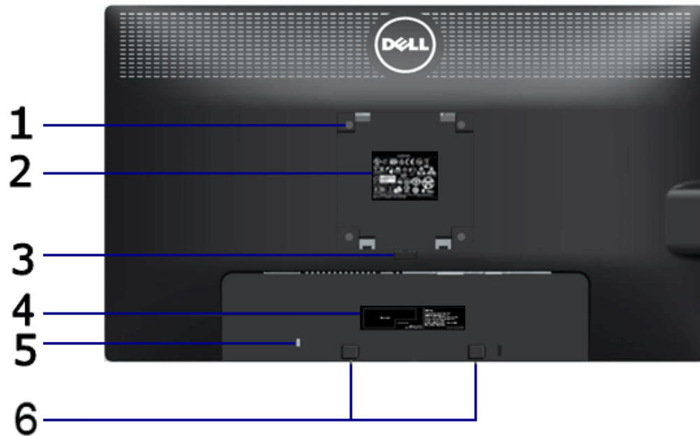
Vista trasera
